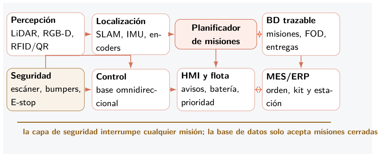
Figura 8.1: Arquitectura propuesta para el Sistema AMR-FOD-Kitting.
