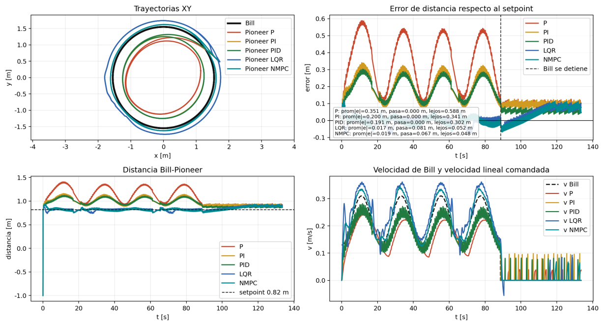
Figura 4.4: Comparación temporal de P, PI, PID, LQR y NMPC en la escena de seguimiento de Bill.
