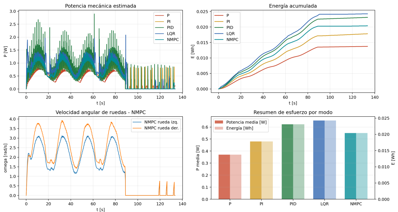
Figura 4.5: Coste físico aproximado del seguidor: potencia instantánea y energía acumulada en las ruedas.
