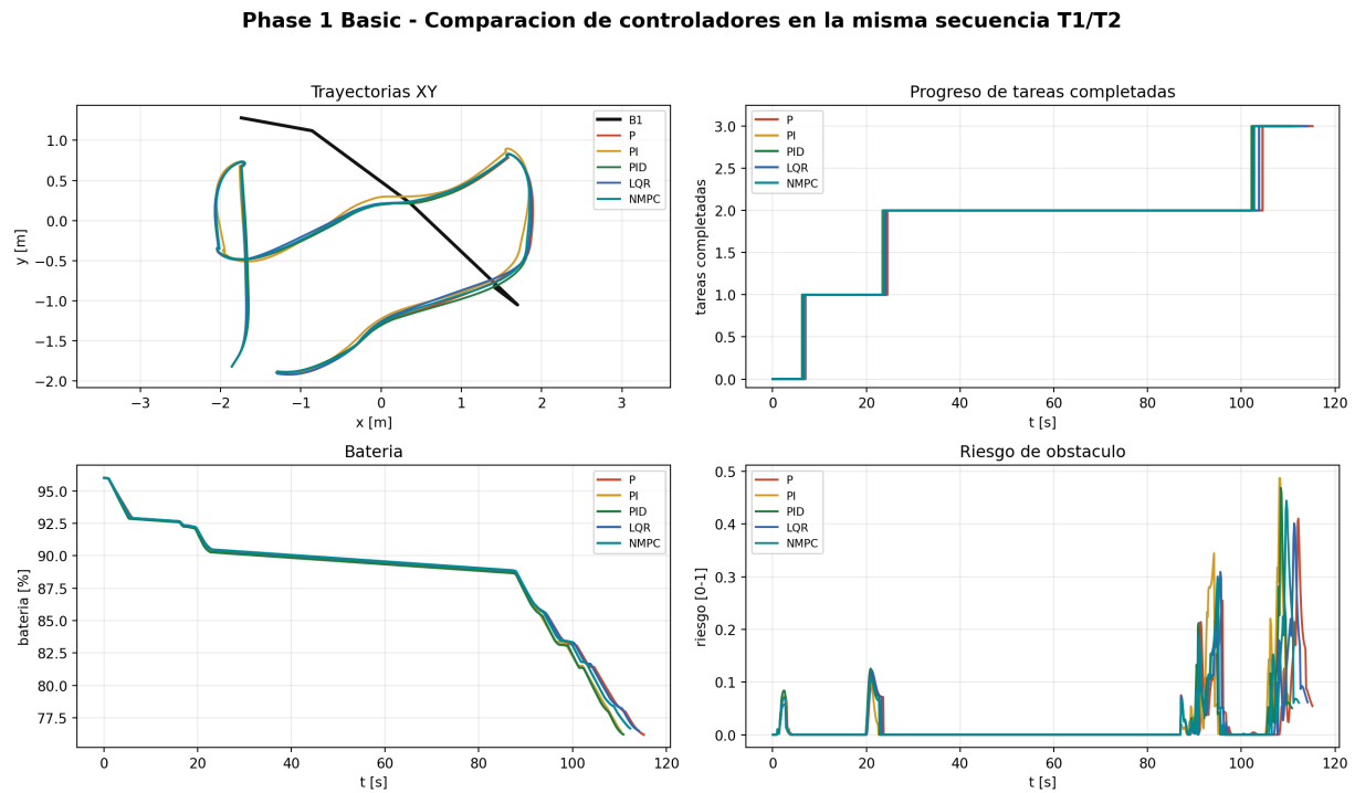
Figura 3.1: Comparación de modos de control exportada desde CoppeliaSim. Todos los modos completan la tarea. PI obtiene el menor puntaje ponderado con los pesos definidos ( n = 1 por modo).
