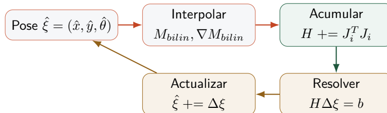
Figura 6.4: Hector SLAM: iteración Gauss-Newton con interpolación bilineal del mapa log-odds. El Hessiano se acumula con los jacobianos analíticos de la transformación rígida; el sistema H \Delta \xi = b se resuelve por la regla de Cramer.
