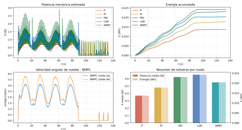
Actividad 2.1 - Datos de ruedas y potencia estimada
