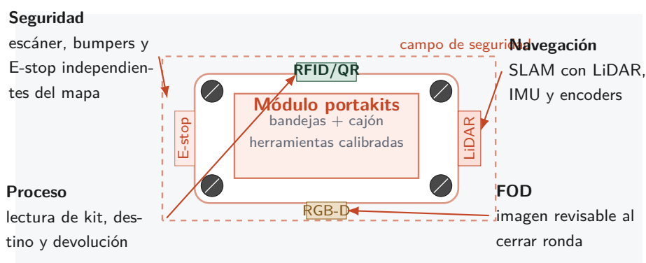
Figura 7.1: Configuración propuesta del AMR-FOD-Kitting.
