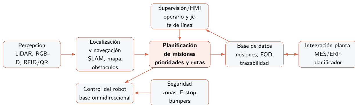
Figura 8.1: Arquitectura propuesta para el Sistema AMR-FOD-Kitting.
