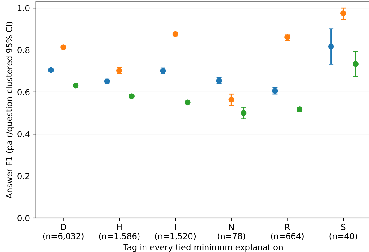
BQA
