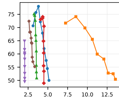
Gilbert-Elliott
