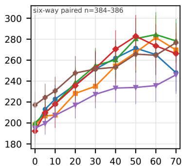
Gilbert-Elliott
