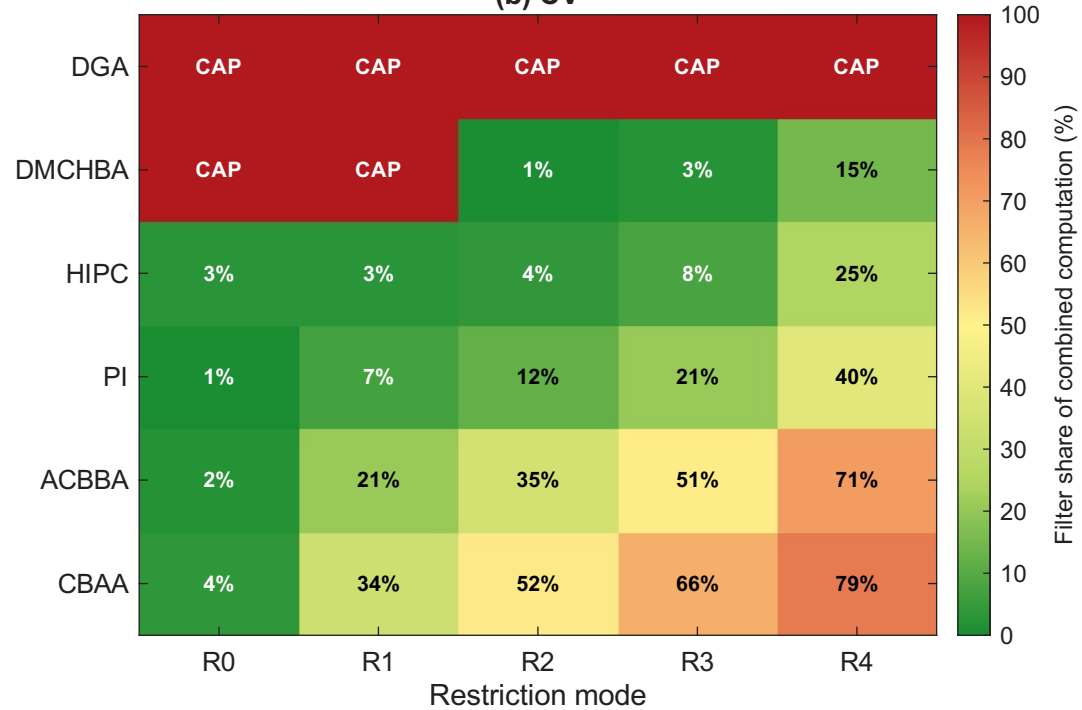
(b) CV
