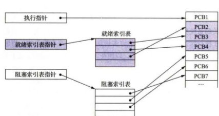
图 2-13 PCB 索引方式示意图
