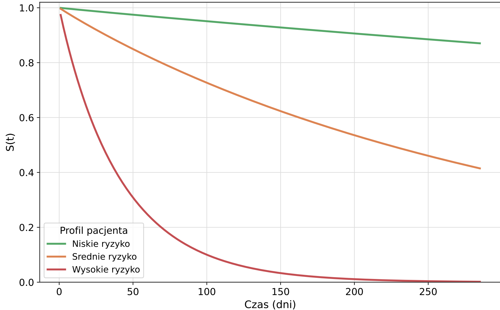
Funkcja przeżycia – Weibull AFT (profile ryzyka)
