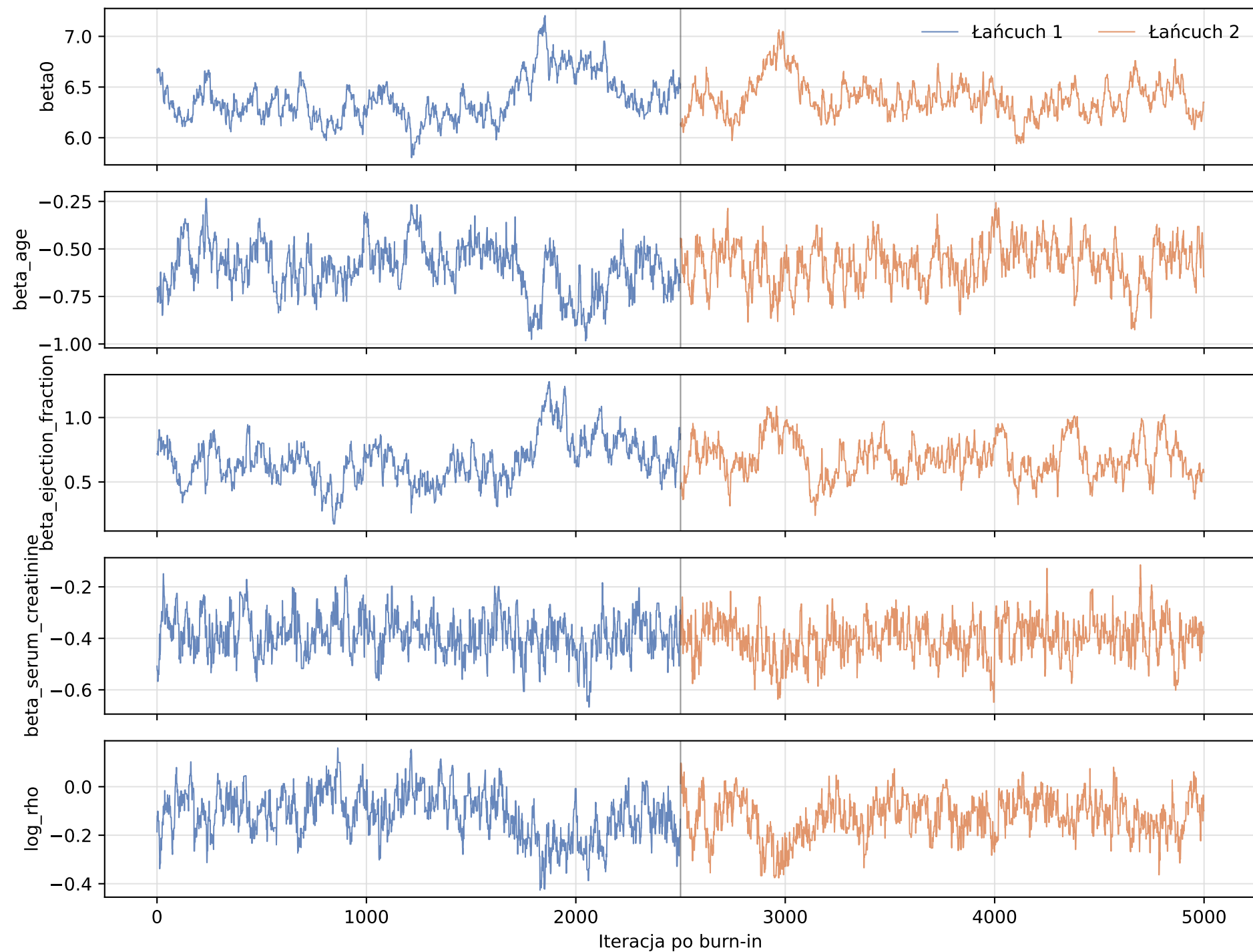
Traceploty MCMC; średnia akceptacja = 0.534
