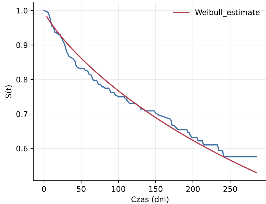
Dopasowanie funkcji przeżycia
