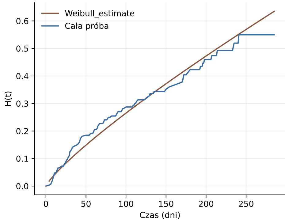
Skumulowany hazard
