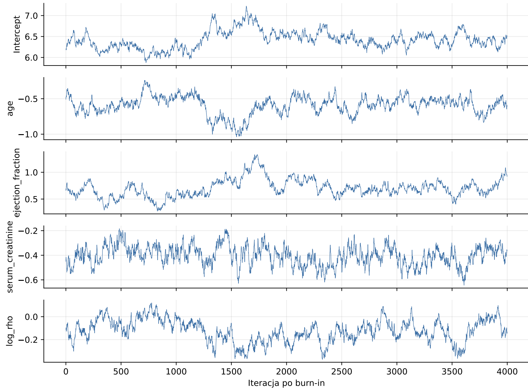
Traceploty MCMC; akceptacja = 0.78
