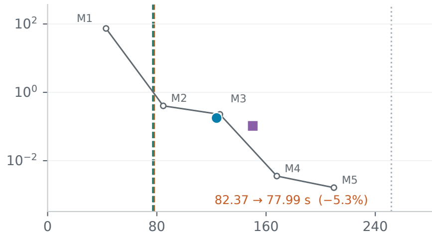
Benjamin-Feir
