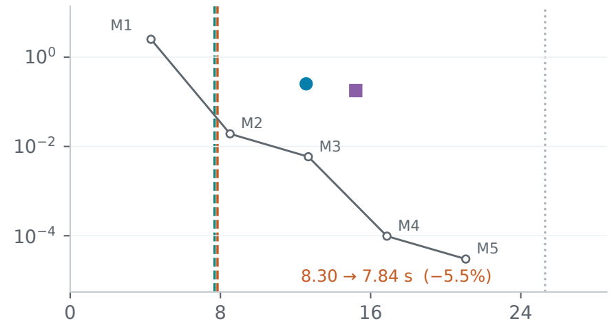
JONSWAP / TMA
