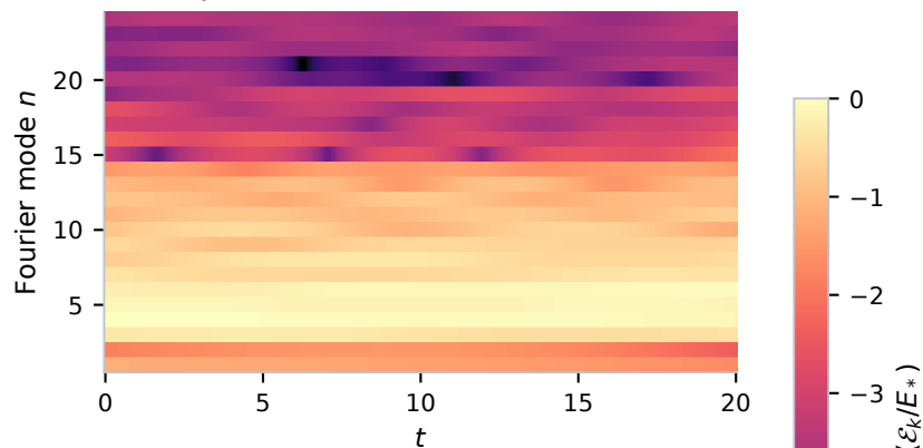
JONSWAP/TMA · C27
