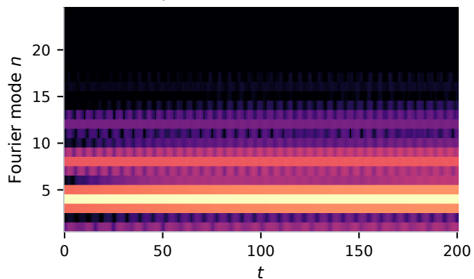
Benjamin-Feir · C27
