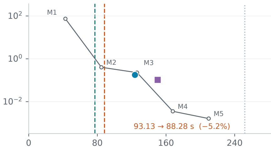
Benjamin-Feir
