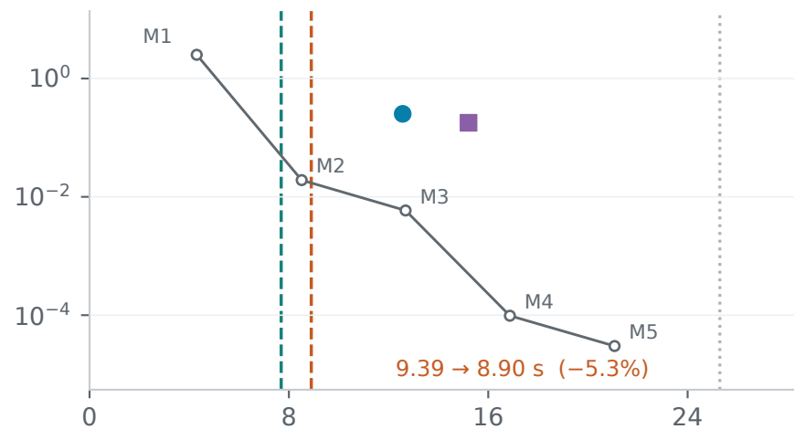
JONSWAP / TMA
