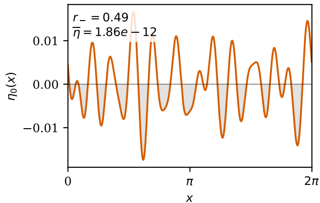
(d) deep-water random sea, case 12: guard inactive
