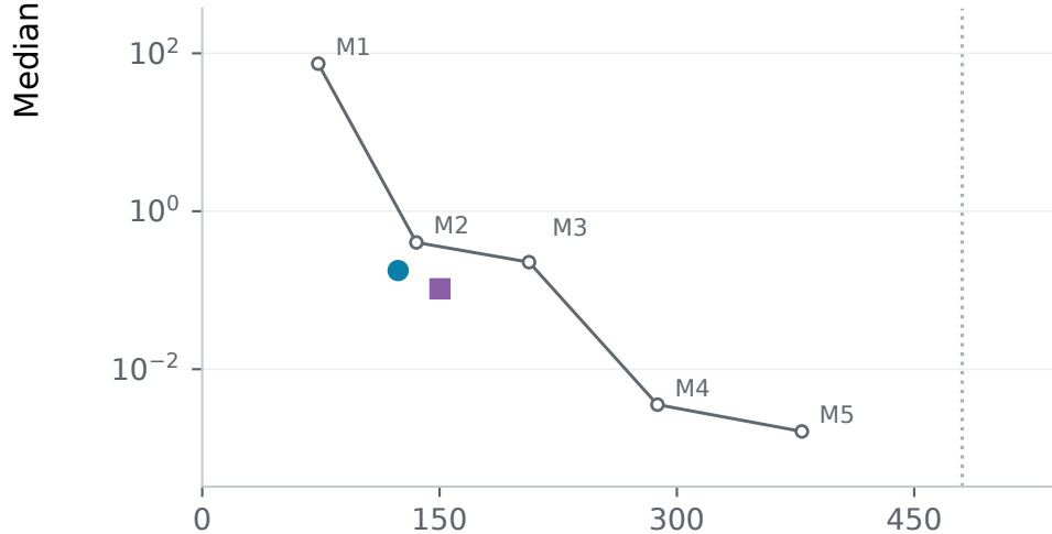
Benjamin-Feir
