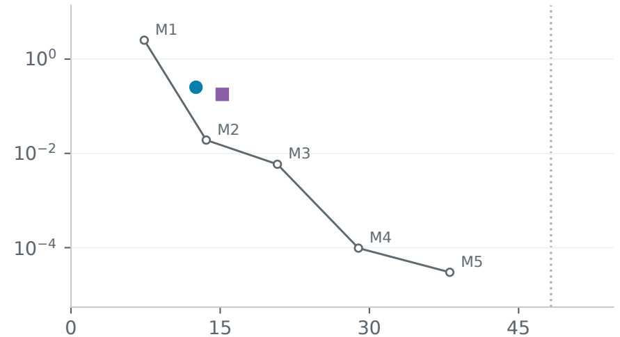
JONSWAP / TMA
