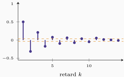
PACF : décroissance
