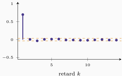
PACF : coupée après k = 1
