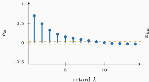
ACF : décroissance géométrique
