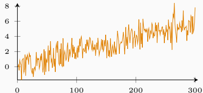
marche aléatoire : \phi = 1
