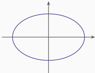
(a) définie positive : Q(x) = 1 est une ellipse
