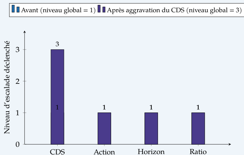
FIG. 2 : Niveau d'escalade déclenché par chacun des quatre indicateurs, avant et après l'aggravation du spread de CDS : seul l'indicateur CDS change, de 1 à 3, ce qui suffit à porter le niveau global (le maximum des quatre) de 1 à 3.
