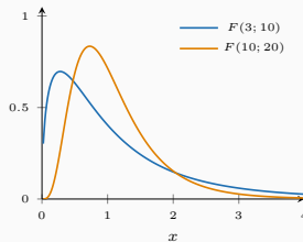
Fisher : un rapport de deux \chi^2
