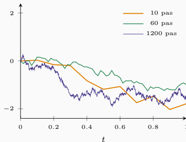
la marche aléatoire, de plus en plus fine
