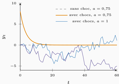
la récurrence perturbée
