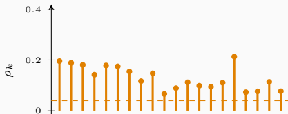
avant : ACF de r_t^2
