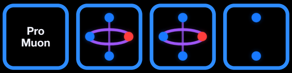
Pro Muon pro-muon
