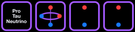
Pro Tau Neutrino pro-tau-neutrino
