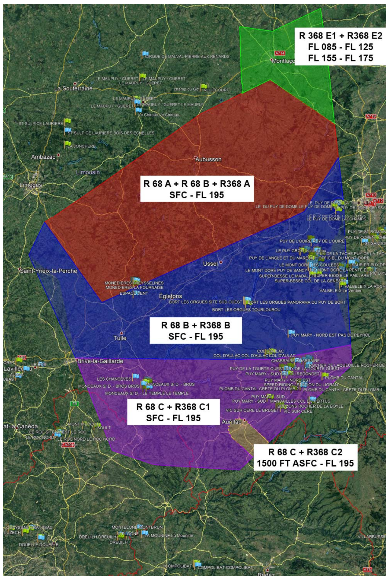
Figure 22. La Zone Centre - Vue d'ensemble
