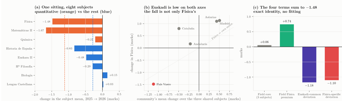
Figura 2: a — las ocho materias vascas, con las tres que las penalizaciones numéricas pueden alcanzar en naranja. b — la variación de Física de cada comunidad frente a su propia media en las tres materias comunes. c — los cuatro términos de la descomposición, que suman el -1.48 observado por construcción.
