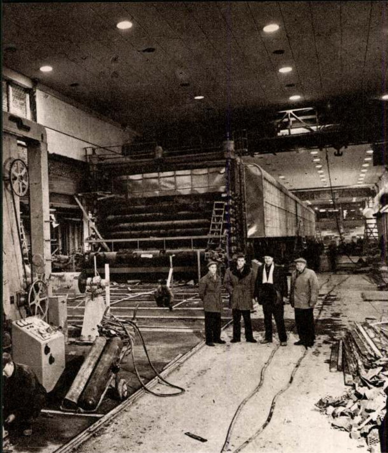
← Koneasentajat Pauli Huhtanen ja Martti Luukkonen rullauskoneen asennuksessa. (etualalla).
