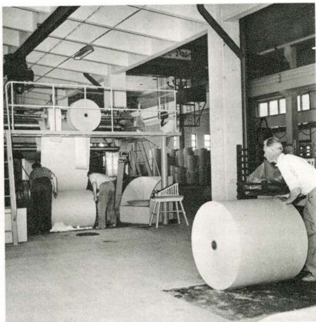
Rullauskoneessa rullataan ja sahataan sanomalehtipaperi määrämittoihin. Rullauskoneen hoitajana on Paavo Peltola ja 1 apumiehenä Tauno Kaaro. ↑
