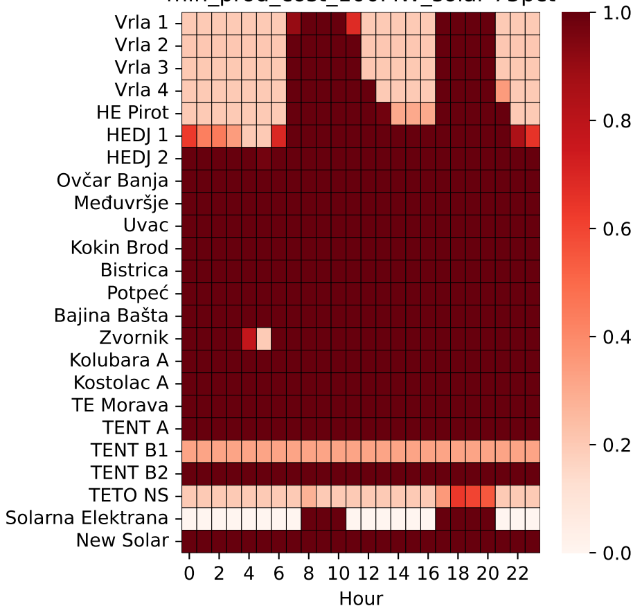
min_prod_cost_100MW_solar-75pct
