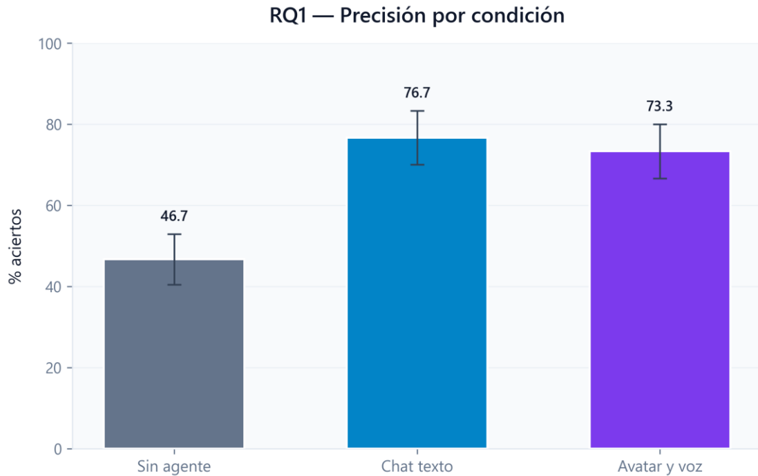
Figura 2. Precisión media por condición
