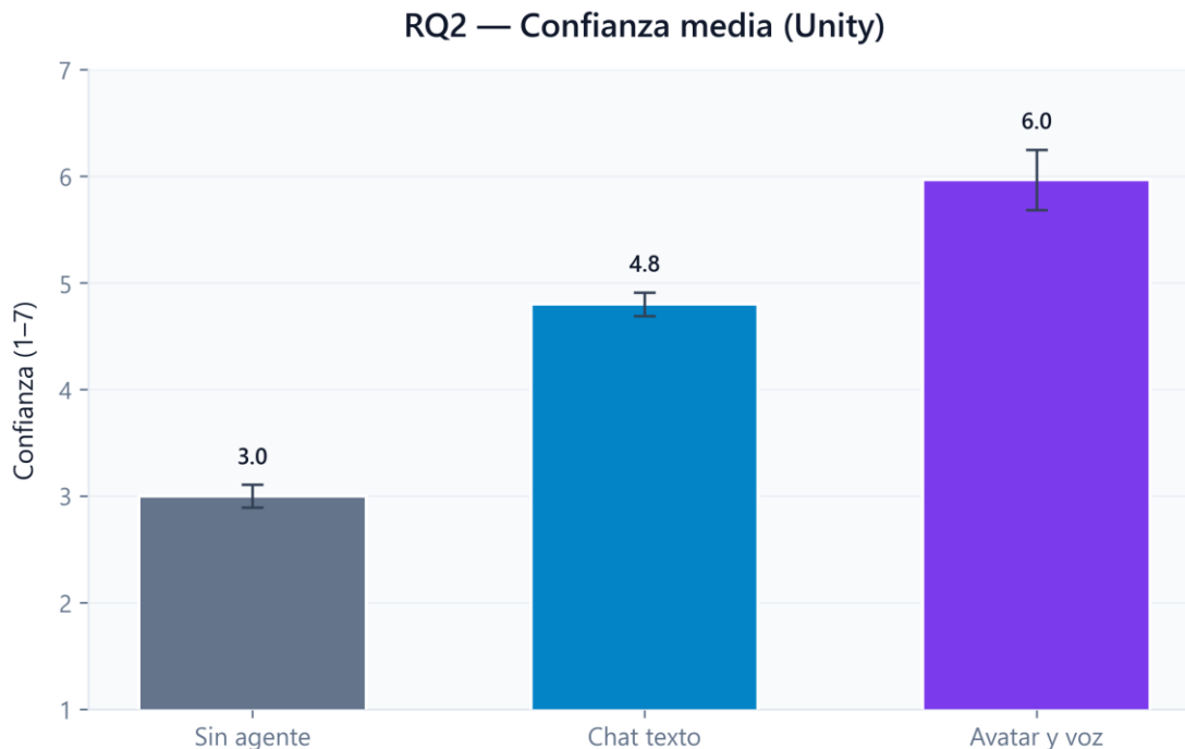
Figura 3. Confianza media por condición
