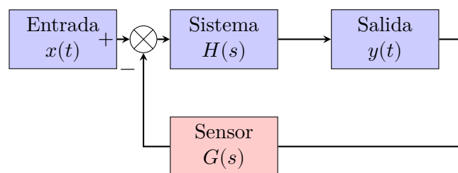
Figura 6.18: Diagrama de bloques de un sistema de control
