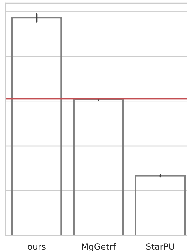
3GPUs
