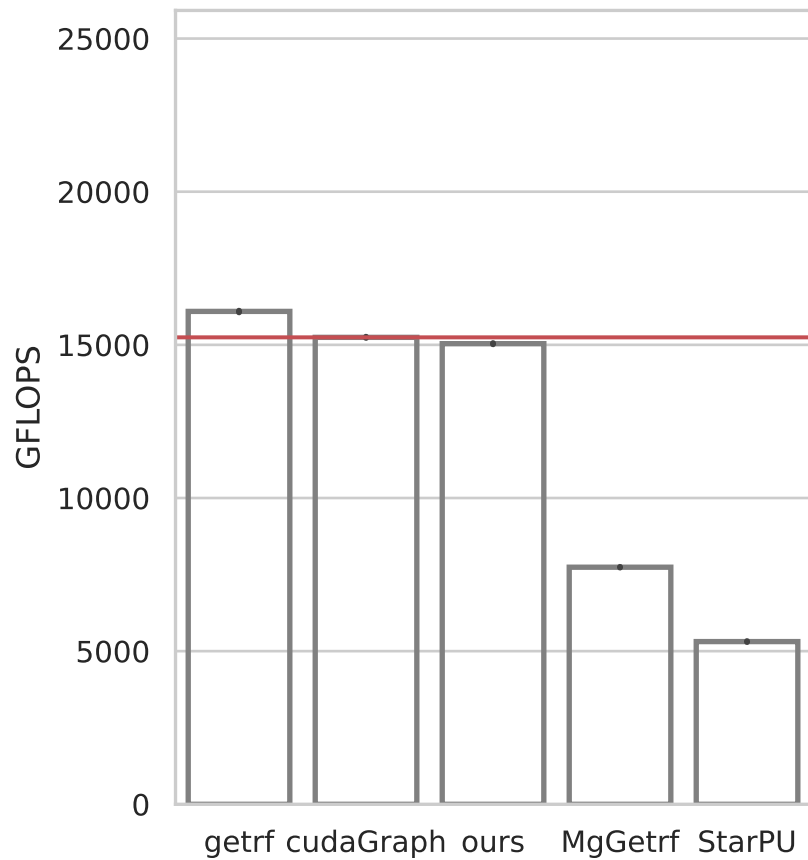
1GPU
