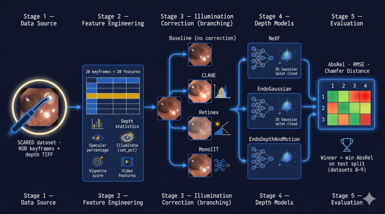
Figura 1. Pipeline del proyecto
