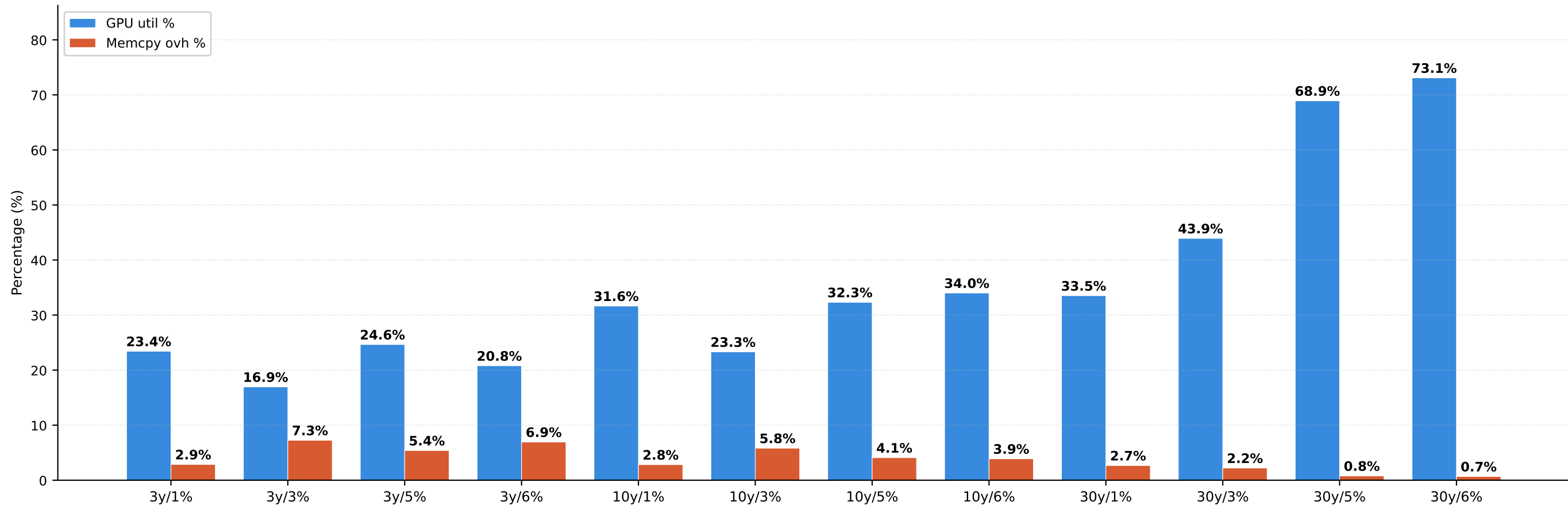
GPU util & memcpy overhead
