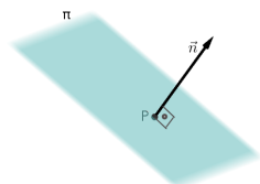
Figura 11: Vector normal a un pla.
