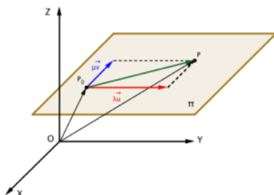
Figura 10: Construcció d'un pla
