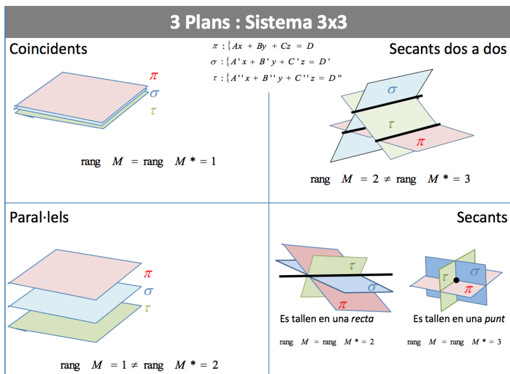
Figura 13: Posició relativa de 3 plans
