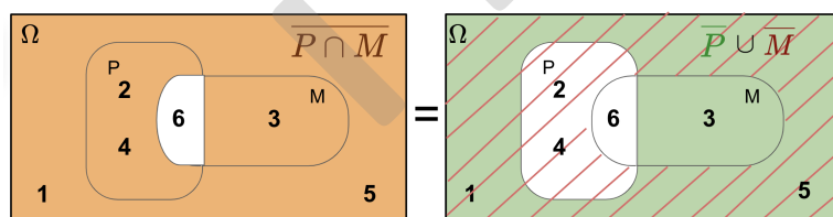
Figura 2: 2a llei de DeMorgan
