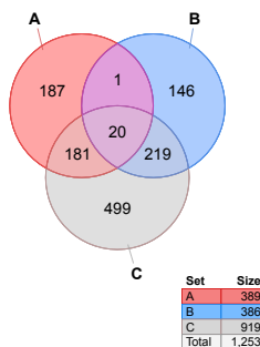
(a) Venn diagram.
