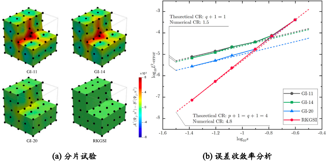
图 7. 伽辽金无网格法误差估计验证
