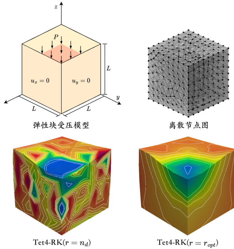
图 4. 免体积自锁有限元-无网格分析方法在弹性块受压问题中的数值验证
