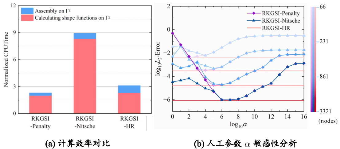
图 5. HR 变分一致型伽辽金无网格本质边界条件施加方案对比传统方案
