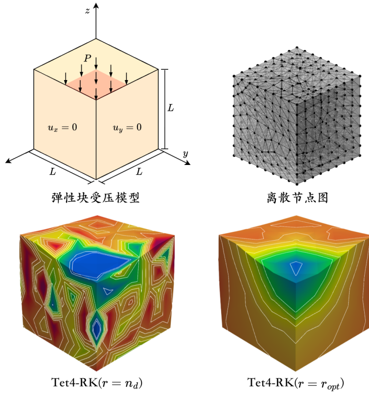
图 3. 免体积自锁有限元-无网格分析方法在弹性块受压问题中的数值验证
