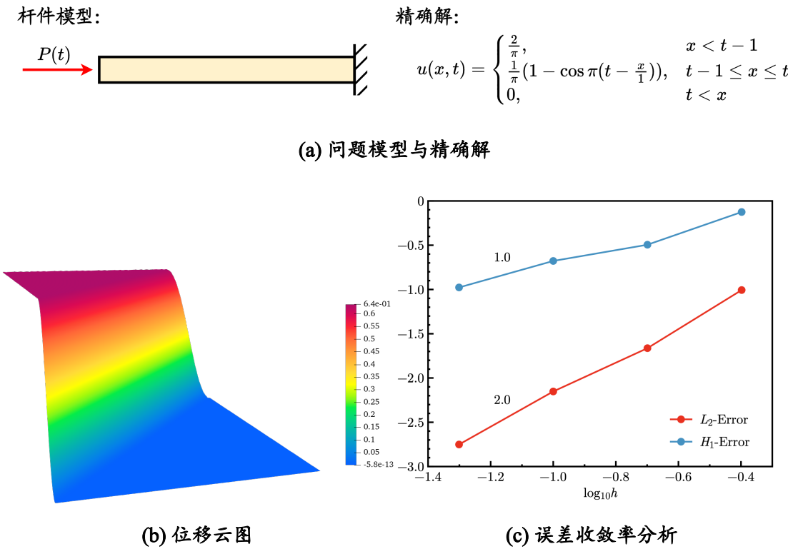
图 6. 拉格朗日型虚位移边界条件施加方案初步测试：杆结构动力问题
