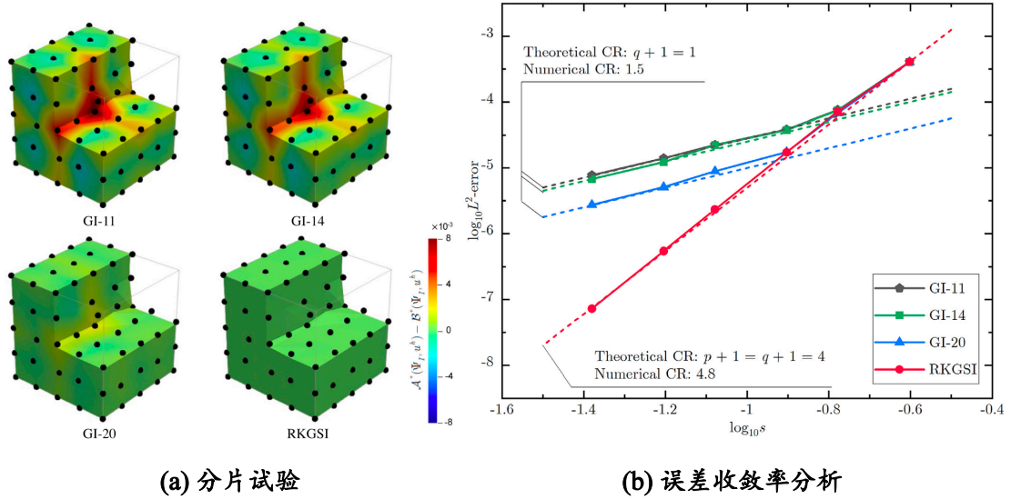
图 5. 伽辽金无网格法误差估计验证
