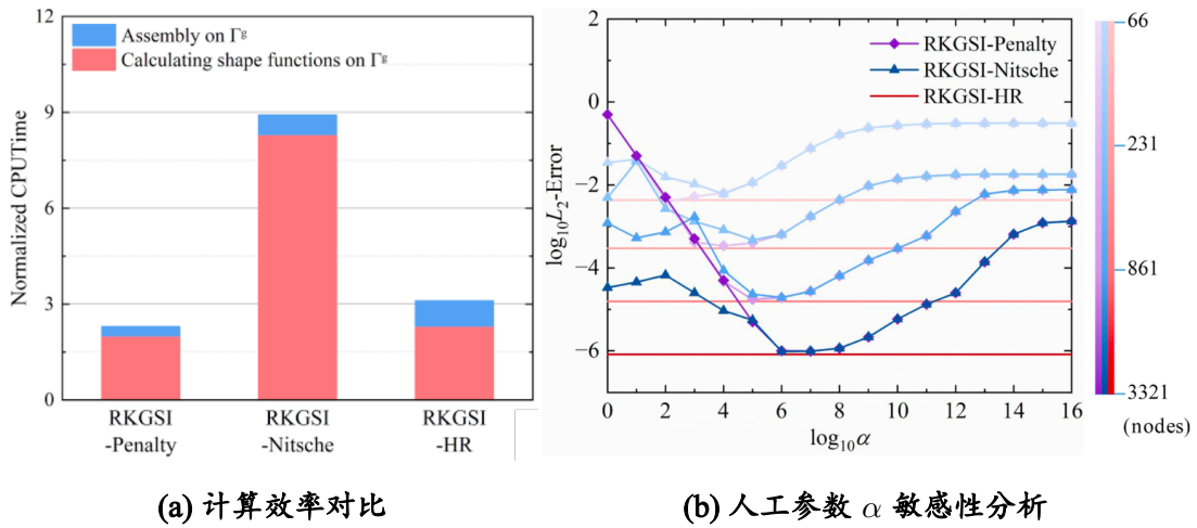
图 3. HR 变分一致型伽辽金无网格本质边界条件施加方案对比传统方案
