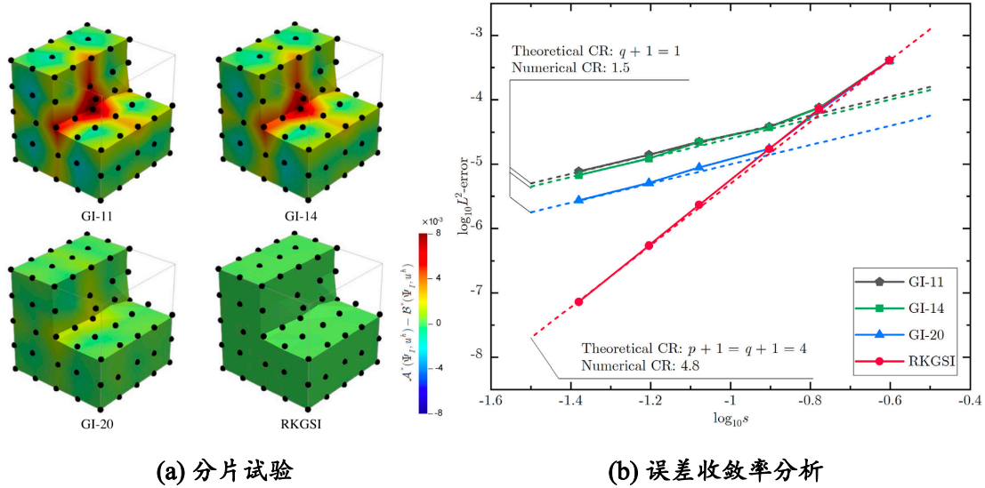
图 4. 伽辽金无网格法误差估计验证
