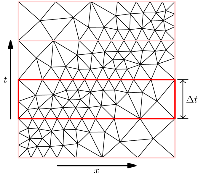
图 1. 时空混合离散间断伽辽金法网格划分
