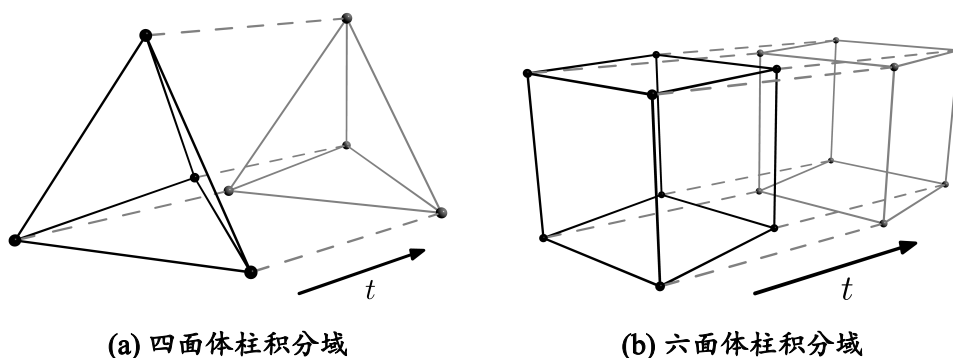
图 3. 四维空间背景积分域
