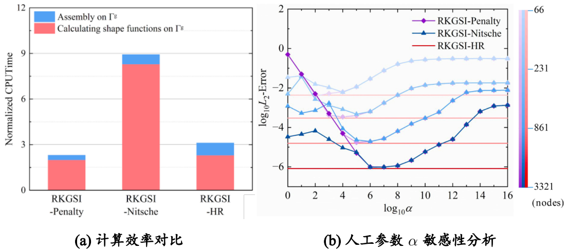
图 2. HR 变分一致型伽辽金无网格本质边界条件施加方案对比传统方案
