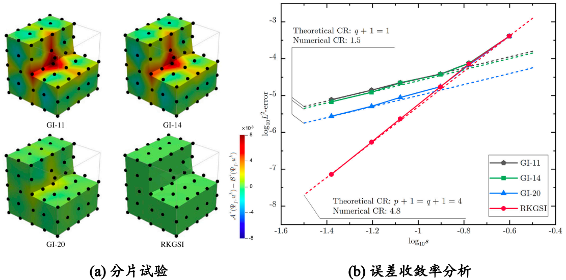
图 3. 伽辽金无网格法误差估计验证
