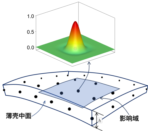
再生核无网格近似
